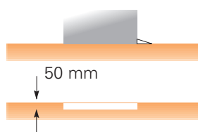
Cibes plattformheiser kan monteres i en 50 mm utsparing eller direkte på gulv med en 50 mm rampe. Det øvre høyre bildet viser heisen i standard utførelse med A1 dør.
