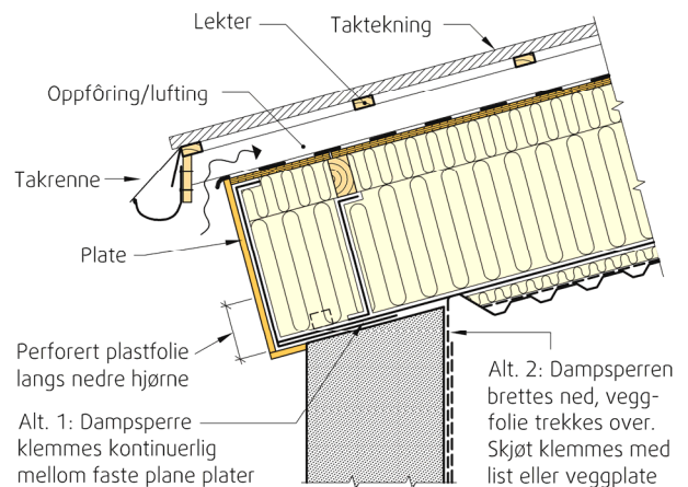
Fig. 4 Prinsipp for utførelse av tilslutning til yttervegg for tak med utvendig nedløp.
